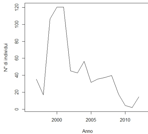
Componente di trend
