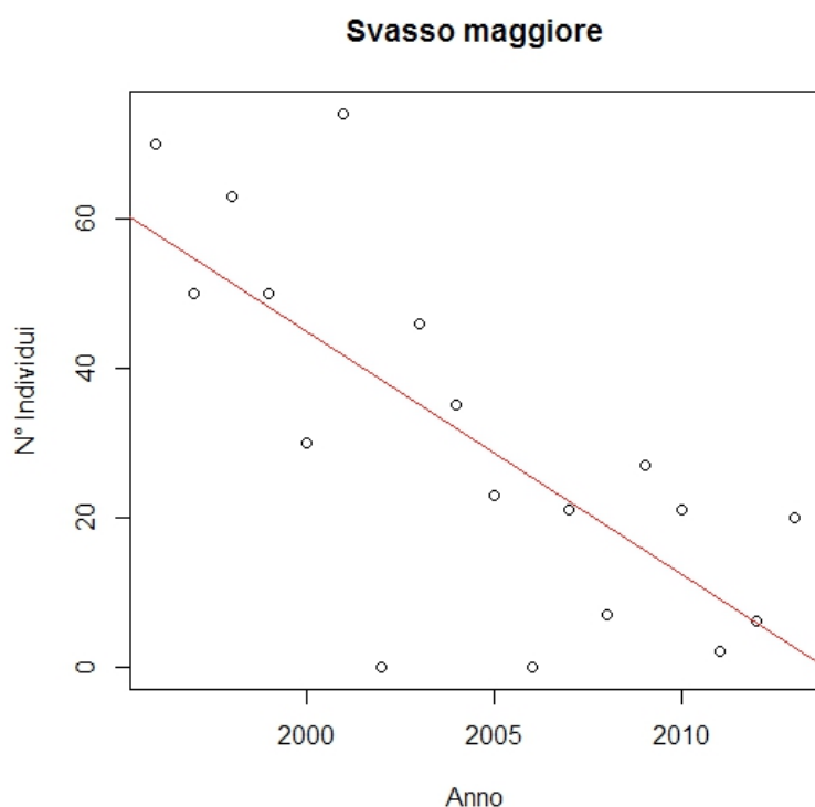
Figura 4 - Modello di regressione semplice.
